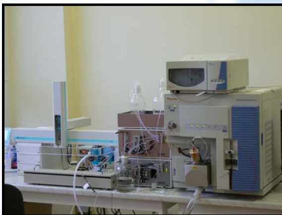
Obr. Kapalinový chromatograf s trojitým kvadrupolovým spektrometrem
